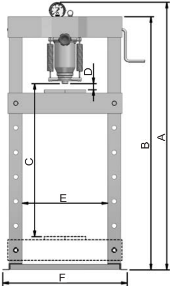
Modelo P15000; P15300; P15200 e P30000
